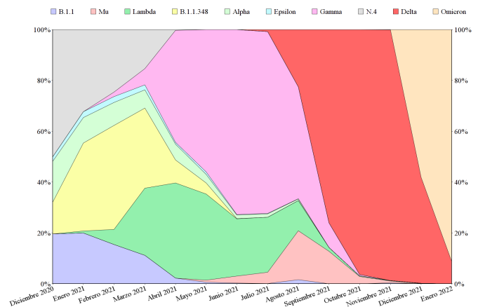
Figura 5: Evolución de los linajes predominantes de SARS-CoV-2 en Chile, diciembre 2020 - 10 de febrero 2022
