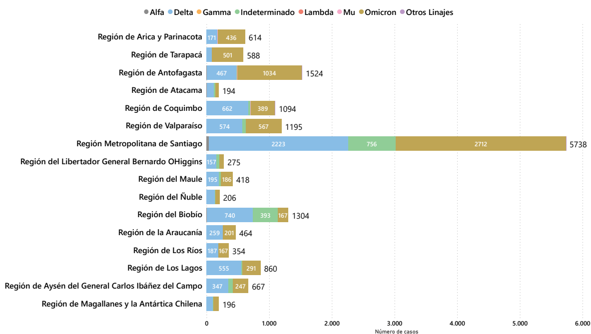
Figura 12: Casos de SARS-CoV-2 en comunitarios secuenciados y genotipificados de variantes y linajes en seguimiento de SARS-CoV-2 según región de residencia. Chile, SE 48 de 2021 a la 05 de 2022 .
