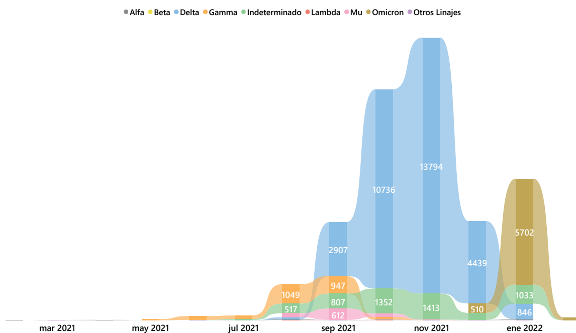
Figura 19: VOC, VOI y linajes principales de casos de SARS-CoV-2 genotipificados según fecha de toma de muestra de test diagnóstico. Chile, 22 diciembre 2020 -07 de febrero de 2022 .
